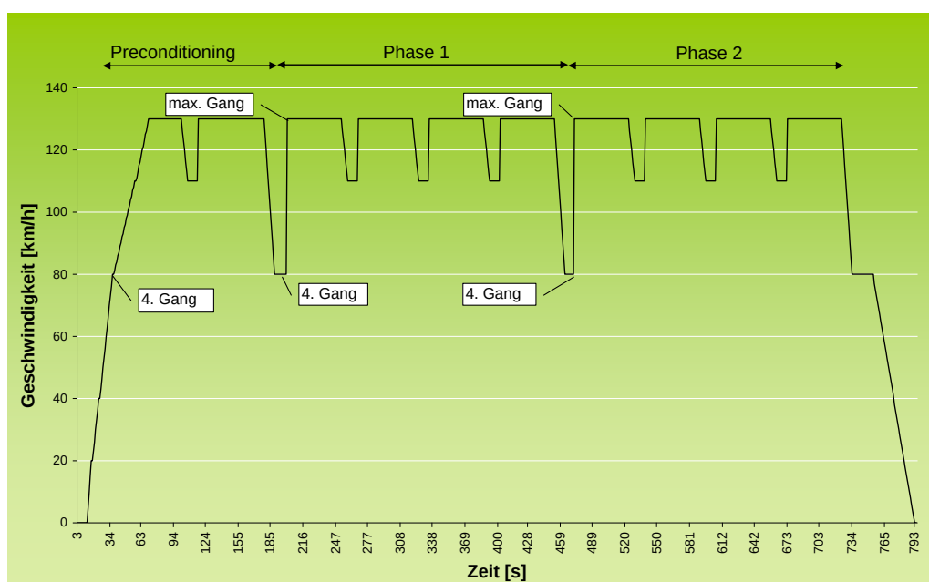
Abbildung 2: ADAC Autobahnzyklus
