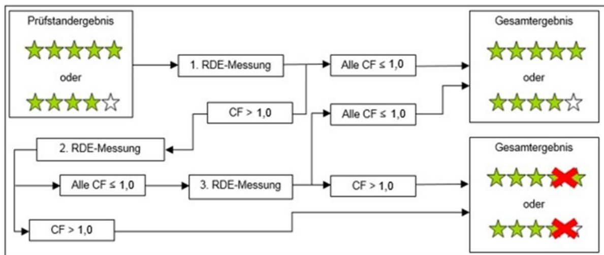
Abbildung 9: Testablauf RDE-Messung
