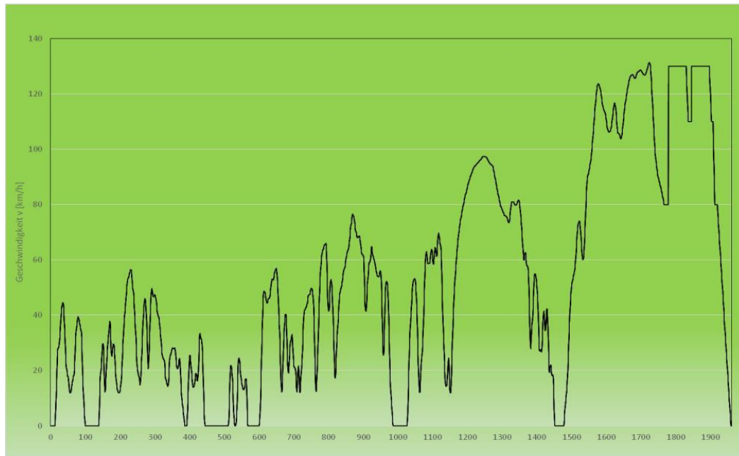
Abbildung 1: ADAC Elektrozyklus
